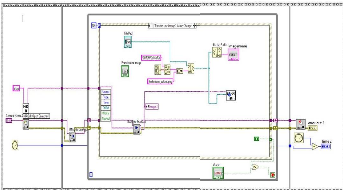
Figure 41 : Block diagramme de capture de défaut
